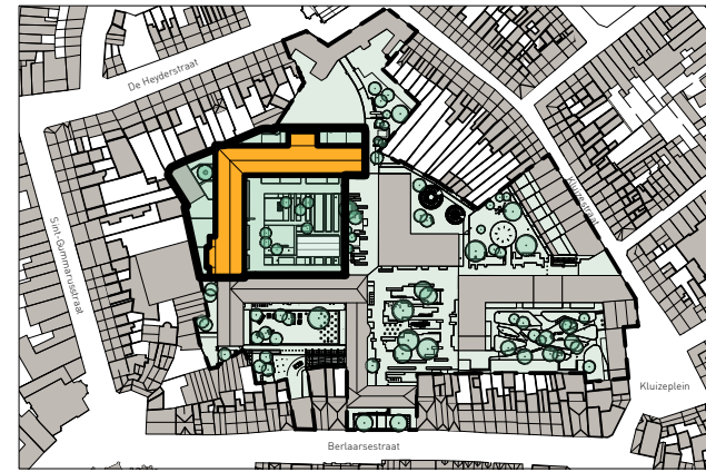
Situering 0 10 20 50 100 m
